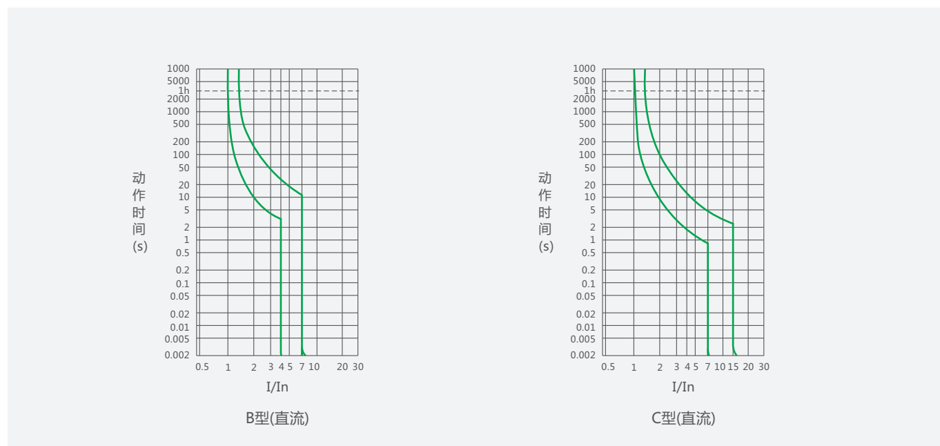
直流脱扣特性曲线
